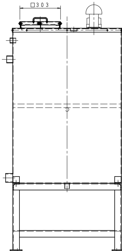
A-A断面
