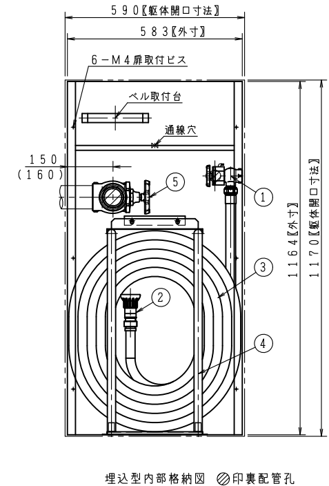
埋込型内部格納図 ⊙印裏配管孔 ( ) 寸法は、露出型
